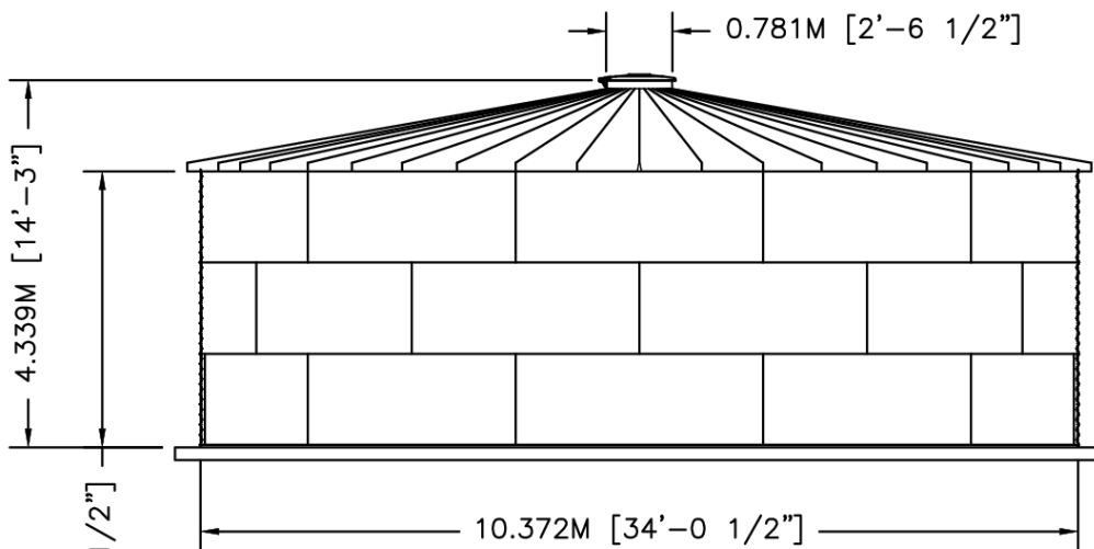
ELEVATION
